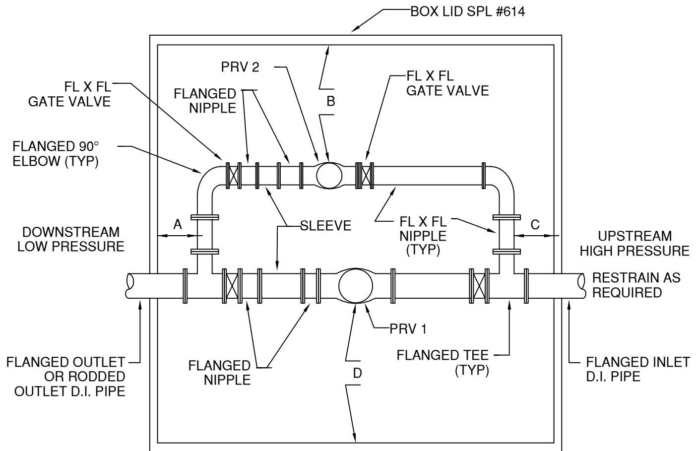
ELEVATION
