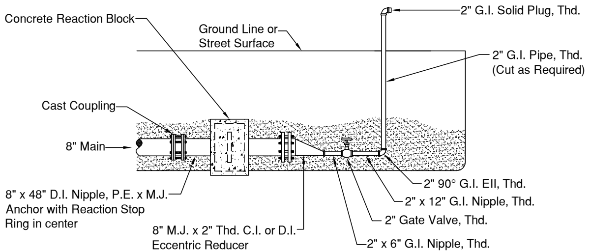
Section A-A
