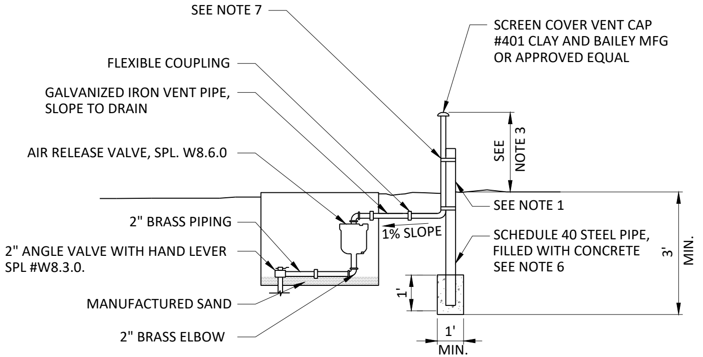
SECTION-A
